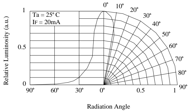
Directivity (Angle : 25°)
