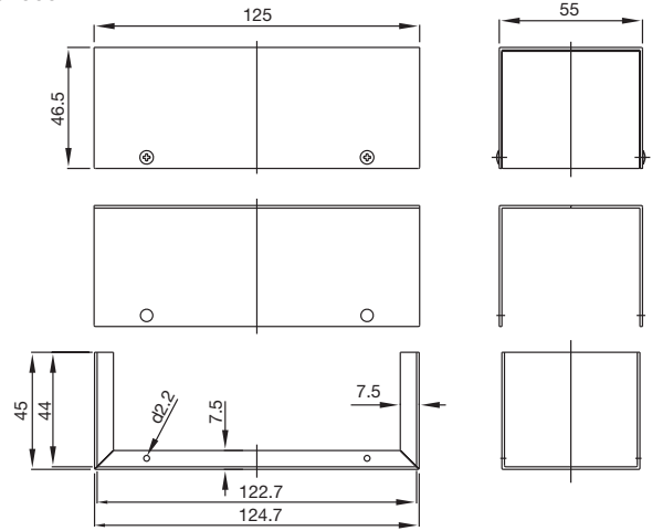
Minibox 31040007
