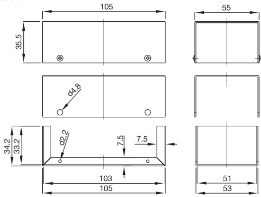
Minibox 31040006
